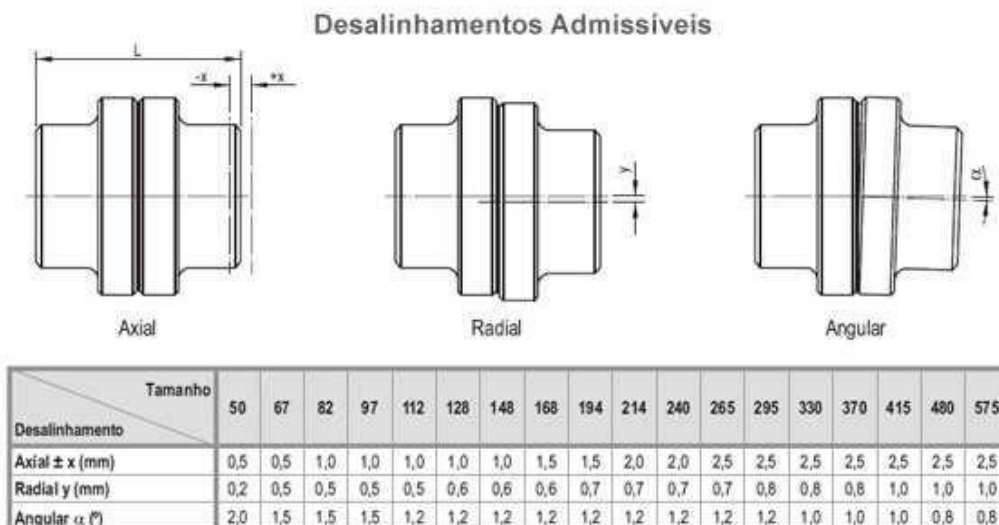
Fig. 16 - Acoplamento elástico convencional
