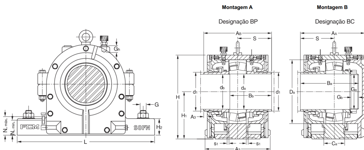
Fig. 25 – Caixa SOFN bipartida com tampas.
