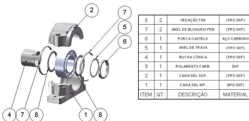
Fig. 23 – Rolamento Conoidal CARB – Axial Livre com anel de bloqueio
