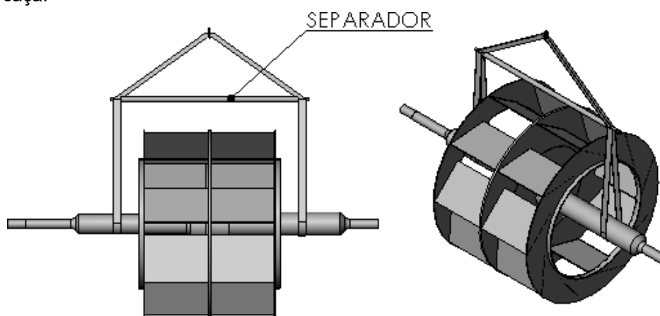
Fig. 5 – Forma de manuseio de rotores duplos
