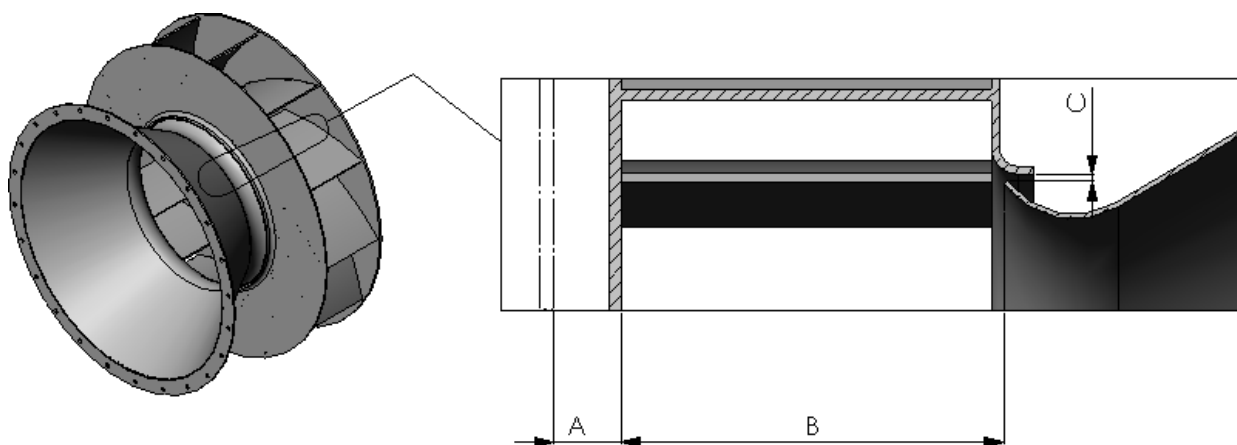
Fig. 12 – Ajustes de cone de entrada e rotor
