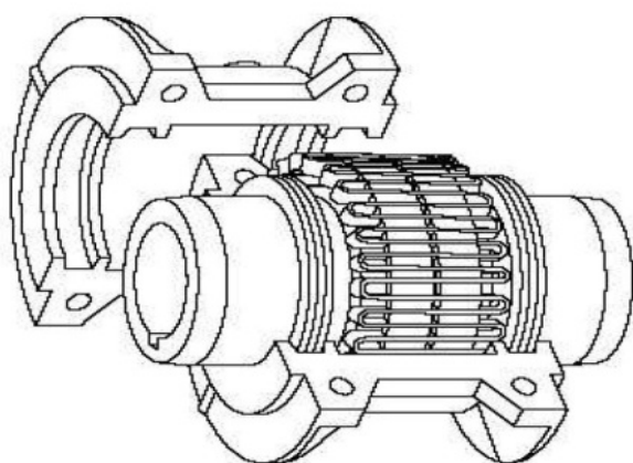
Fig. 17 - Acoplamento de grade elástica
