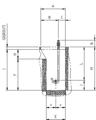
Fig. 7 - Chumbador gancho de ancoragem
