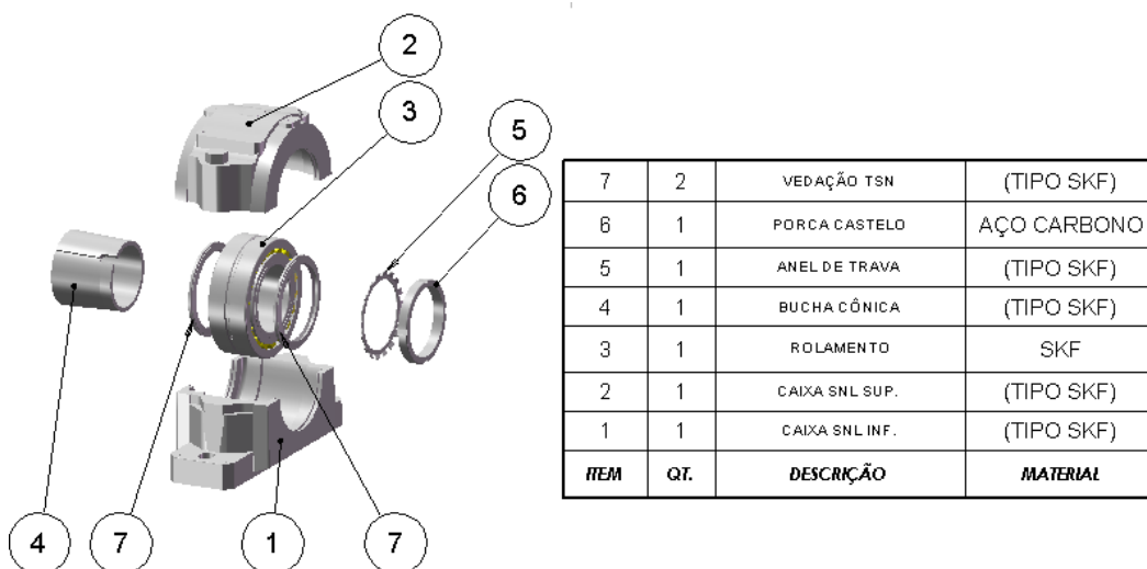
Fig. 22 – Rolamento Autocompensador – Livre
