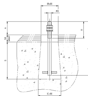
Fig. 8 - Chumbador tirante
