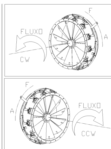
Fig. 14 – Sentido palhetas registro radial
