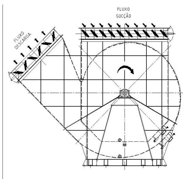
Fig. 13 – Sentido das palhetas registro retangular
