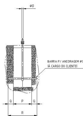
Fig. 7 - Chumbador gancho de ancoragem
