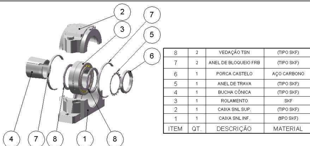
Fig. 21 – Rolamento Autocompensador – Bloqueado
