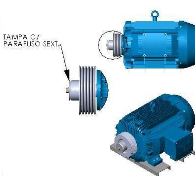
Fig. 19 – Eixo mais curto que polia
