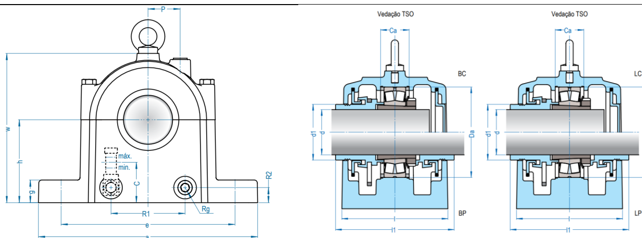
Fig. 24 – Caixa SONL bipartida sem tampas.
