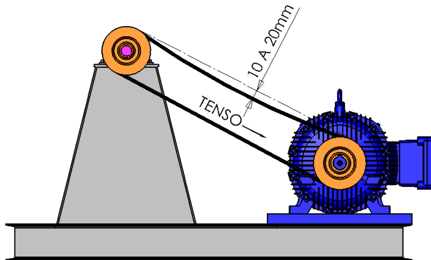
Fig. 20 – Ajuste de tensão na correia
